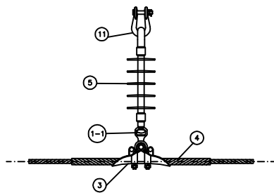
CON PREFORMADO (ARMOR ROD)
