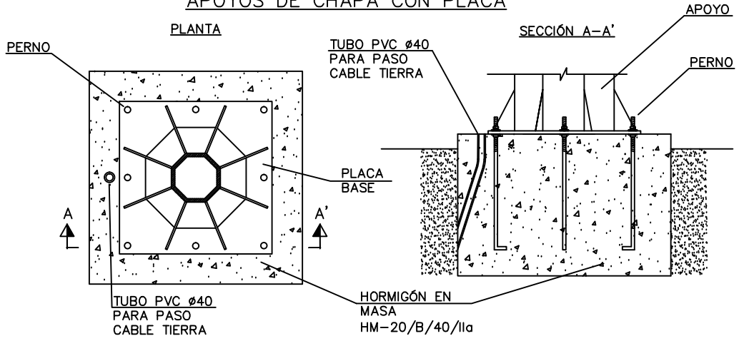
APOYOS DE CHAPA CON PLACA
