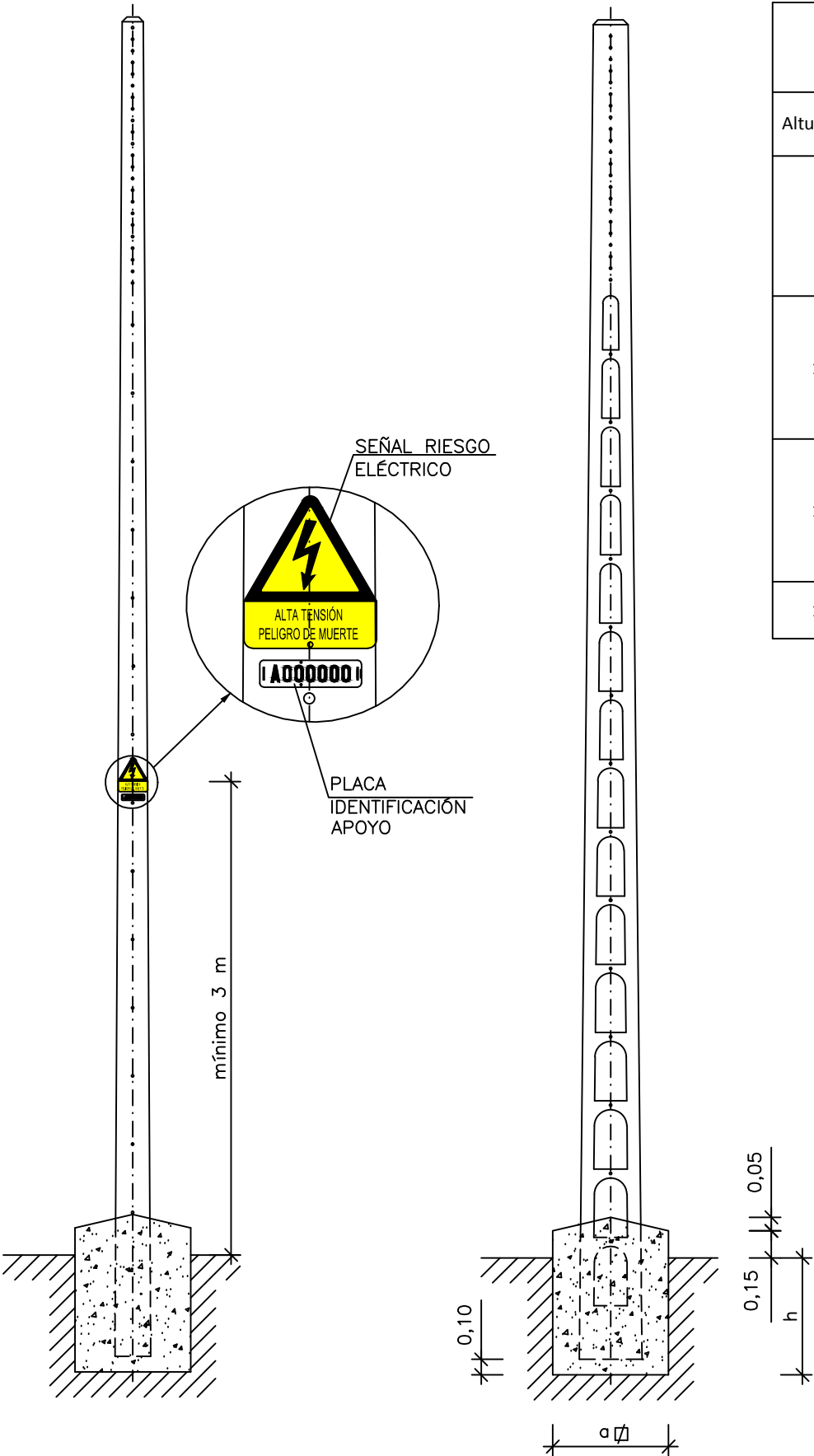
COTAS EN m
