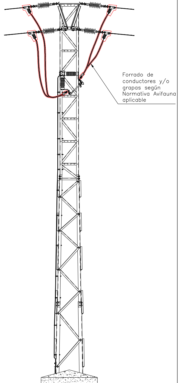
VISTA LATERAL
