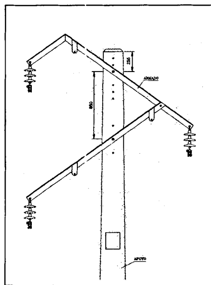
Fig. 5.3.7-D Armado tipo canadiense
