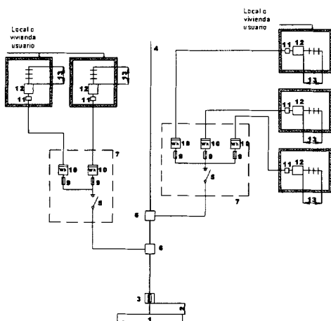
(Esquema 3.3.2.3 Para varios usuarios con contadores en forma centralizada en más de un lugar)
