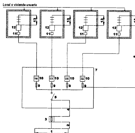
Esquema 3.3.2.2.2. Para varios usuarios con contadores en forma centralizada en un lugar)
